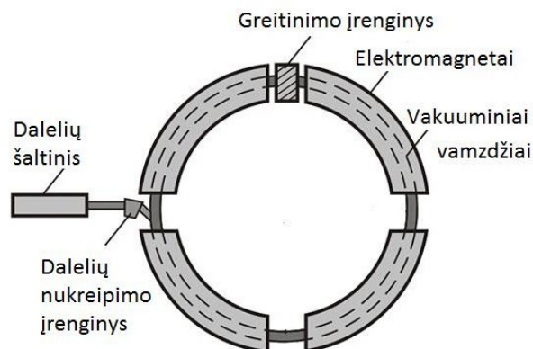
6 pav. Sinchrotrono schema.
