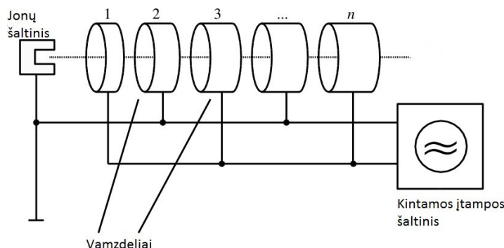
1 pav. Tiesinio pakopinio greitintuvo schema.
